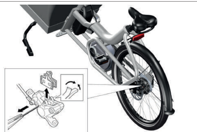
Image 38 : Retrait des plaquettes de frein afin de vérifier leur état d'usure
