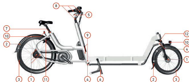
Abbildung 14: Schnelle Sicherheitsprüfung
