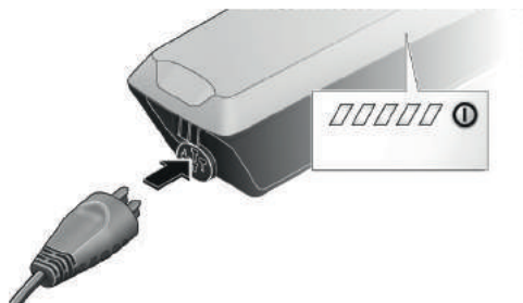
Abbildung 30: Ladegerätstecker in die Ladebuchse am Akku stecken.
