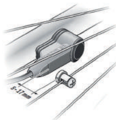
Abbildung 32: Abstand zwischen dem Geschwindigkeitssensor und dem Geschwindigkeitssensormagneten
