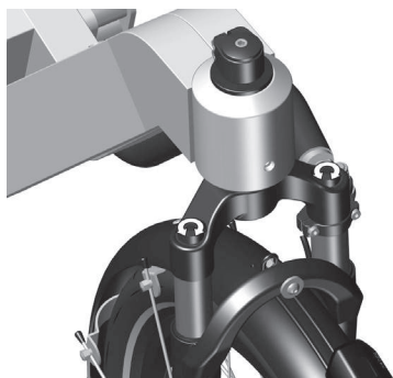
Abbildung 43: Einstellung der Federung
