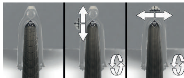
Abbildung 34: Prüfen des Seitenschlags
