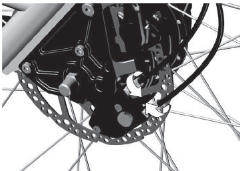
Afbeelding 42: Uitlijning van de markering op de draaigreep (Rohloff versnelling)
