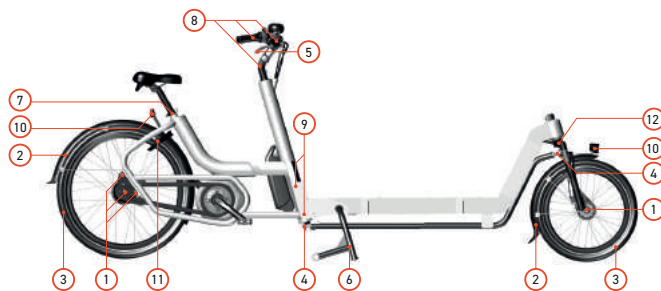
Afbeelding 14: Snelle veiligheidscontrole
