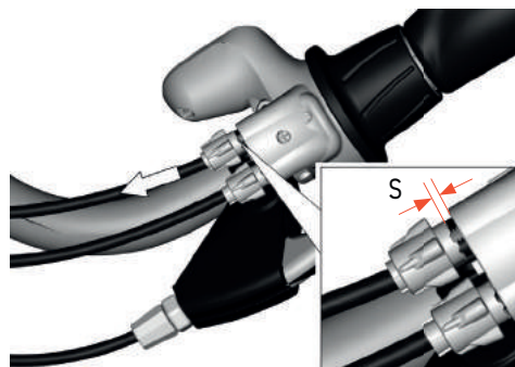
Afbeelding 39: Kabelspeling controleren
