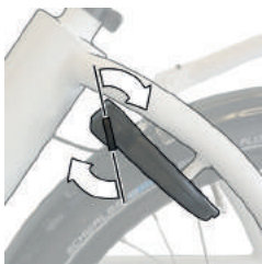
Image 26 : Tournez la clé de 20 à 30 degrés dans le sens des aiguilles d'une montre
