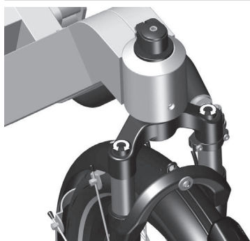
Image 43 : Ajustement du réglage de la suspension
