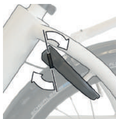
Abbildung 26: Drehen Sie den Schlüssel um 20 bis 30 Grad im Uhrzeigersinn.
